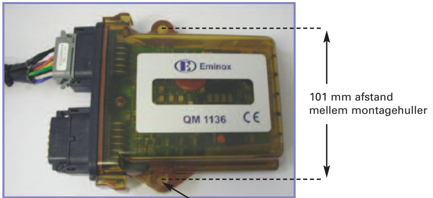
Figur 7. CPU montagehuller
